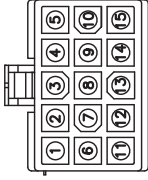
15 pole plug (AMP 172171-1)
